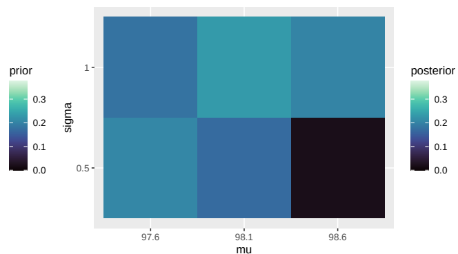
(b) Posterior distribution.
